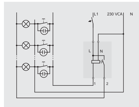
FIG 16.3 CIRCUITO TRIFILAR (TRÊS FIOS)
