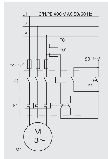
Fig. 9.1.4 ESQUEMA ELÉTRICO
