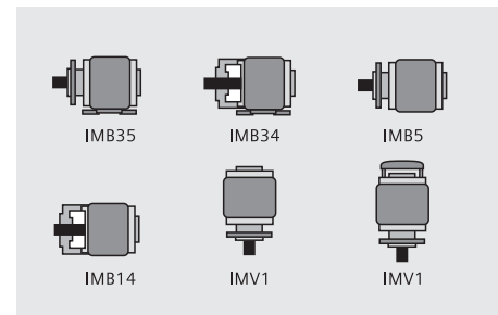
FIG 1.3 POSIÇÕES DE MONTAGEM
