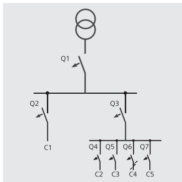
FIG 3.6 SELETIVIDADE RADIAL
