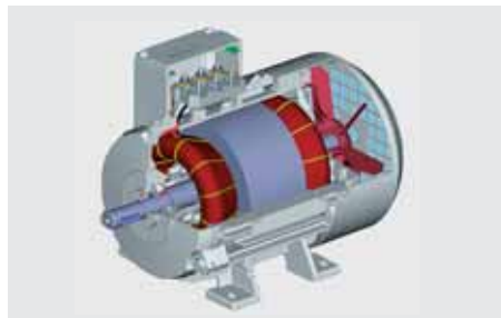
FIG 1.1 CORTE DE UM MOTOR TRIFÁSICO
