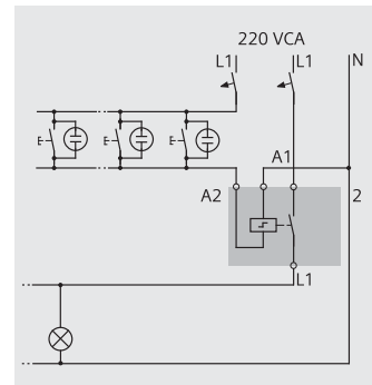
FIG 16.1 CIRCUITO MONOFÁSICO DE ILUMINAÇÃO EM 220 VCVCA
