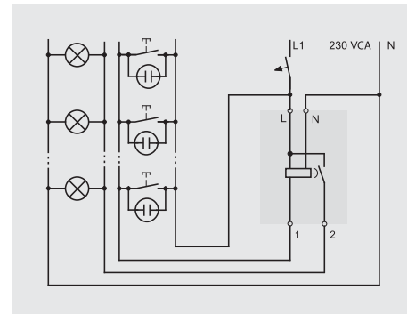
FIG 16.2 CIRCUITO TETRAFILAR (QUATRO FIOS)
