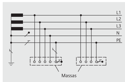
FIG. 2 ESQUEMA TN-S
