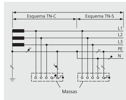
FIG. 3 ESQUEMA TN-C-S
